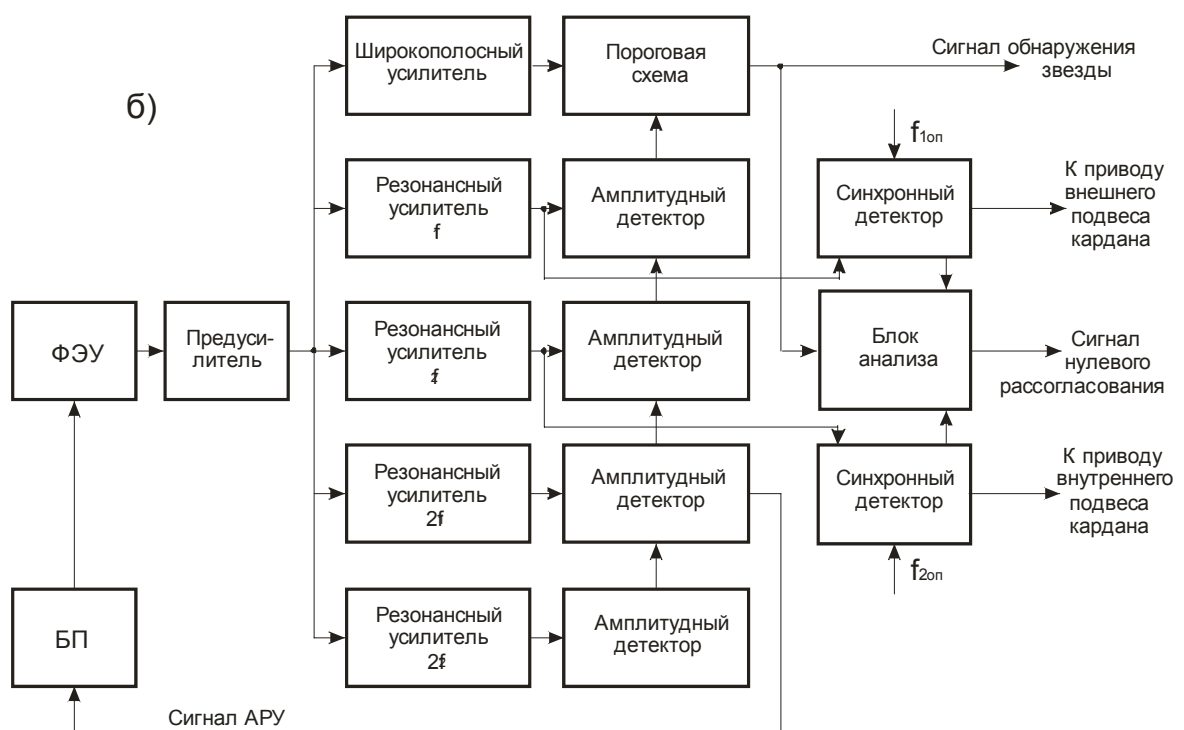
Система ориентации по звездам (астрогид)
