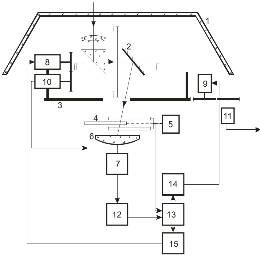
Система ориентации по звездам (секстант)
